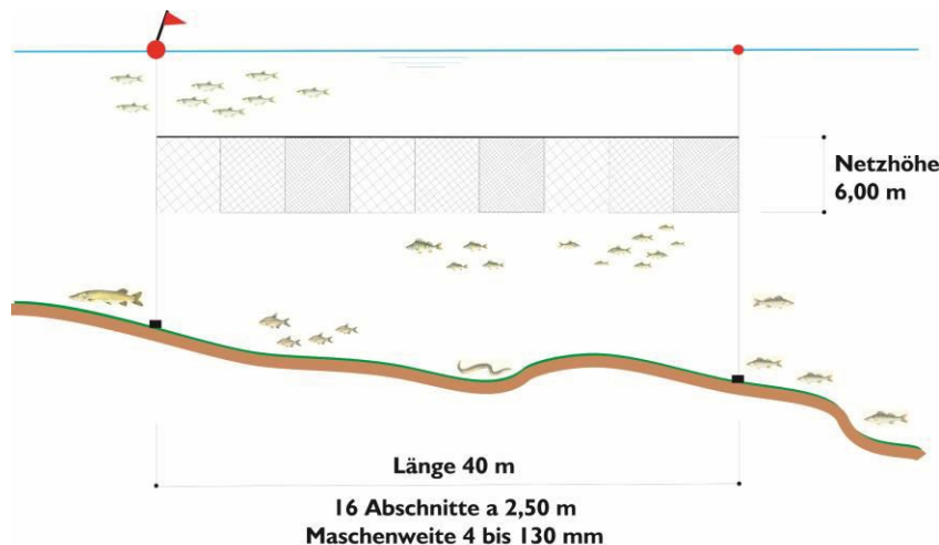
Bild 2: Pelagisches Multimeshnetz
